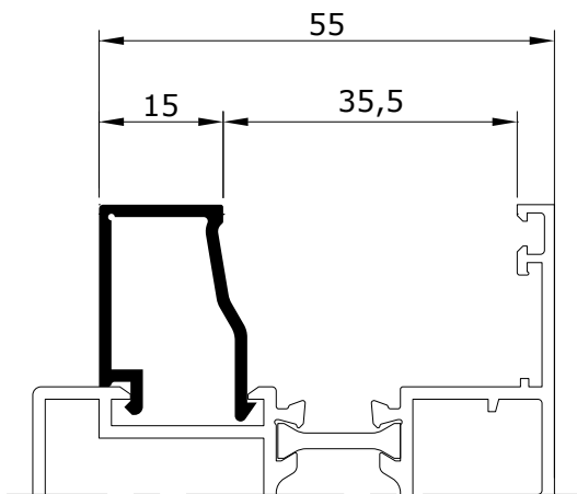
EX 50015-15 0.282 kg/m
