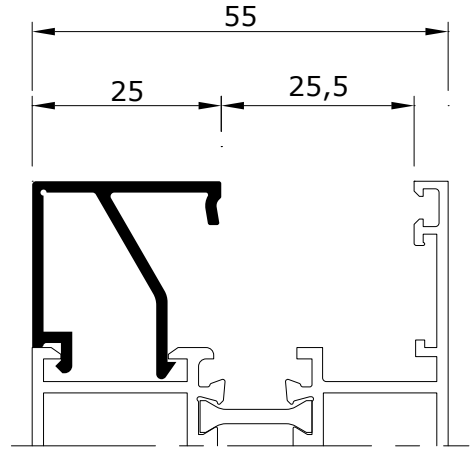
EX 50025-15 0.346 kg/m
