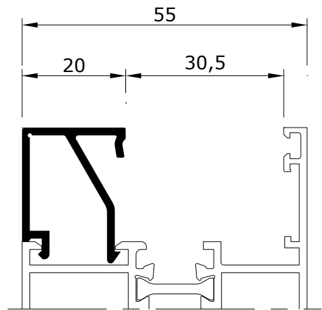
EX 50020-15 0.326 kg/m
