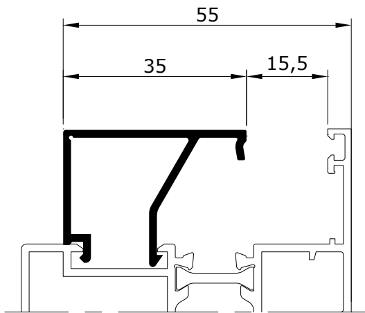
EX 50035-15 0.387 kg/m
