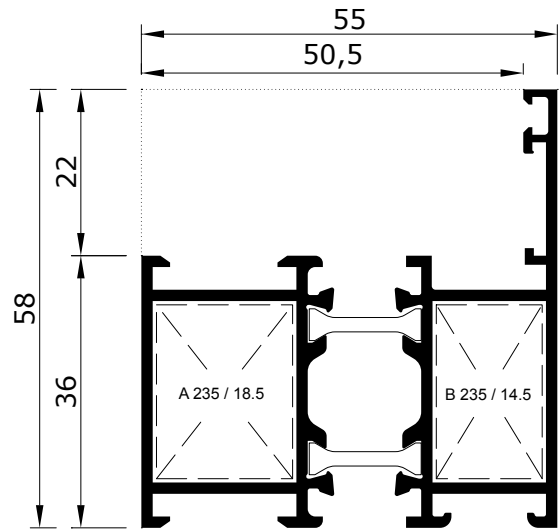
EX-55 10058-15
