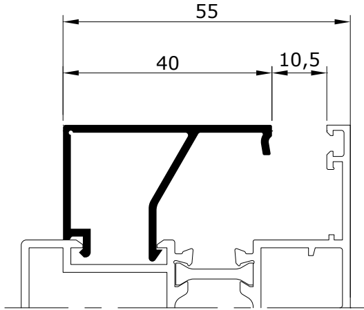
EX 50040-15 0.407 kg/m
