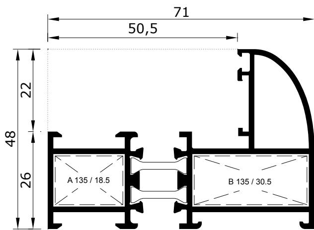
EX-55 14048-15
