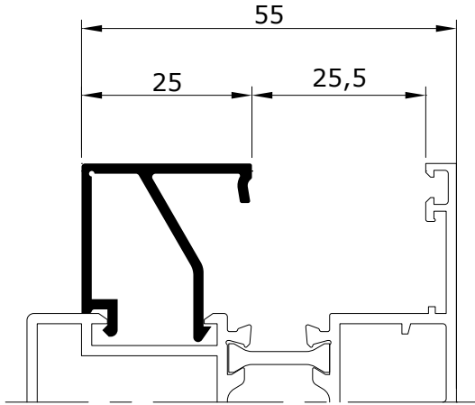
EX 50025-15 0.346 kg/m
