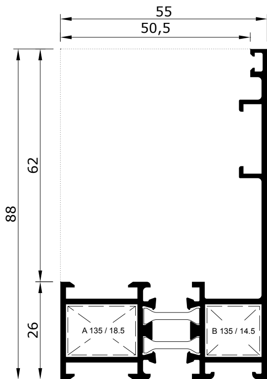
EX-55 12088-15
