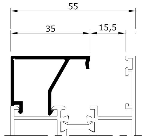
EX 50035-15 0.387 kg/m
