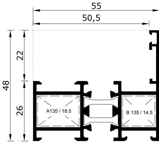
EX-55 10048-15
