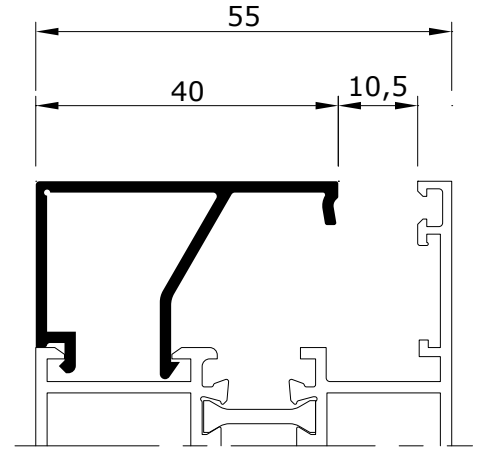
EX 50040-15 0.407 kg/m
