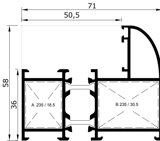
EX-55 14058-15
