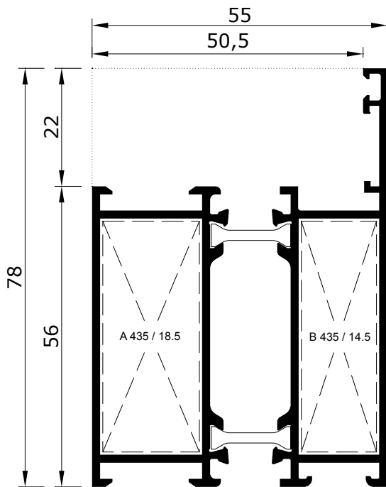
EX-55 10078-15
