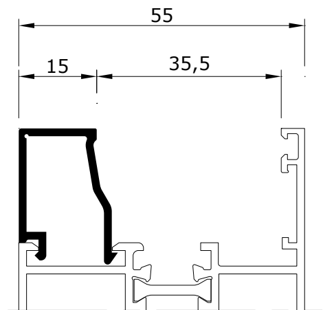
EX 50015-15 0.282 kg/m
