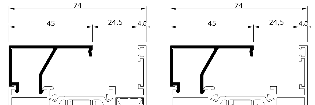
EX 50045-15 0.409 kg/m
