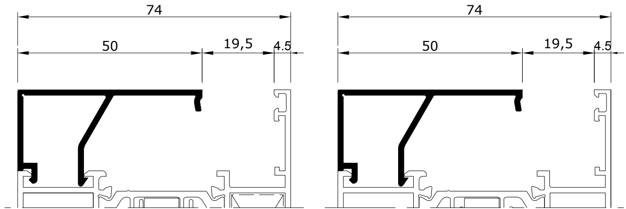
EX 50050-15 0.448 kg/m
