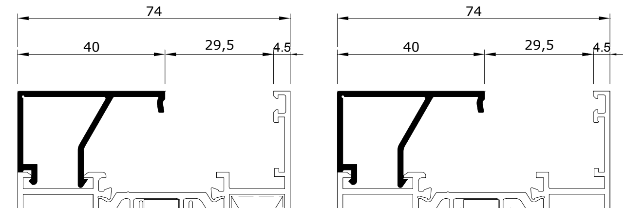
EX 50040-15 0.407 kg/m
