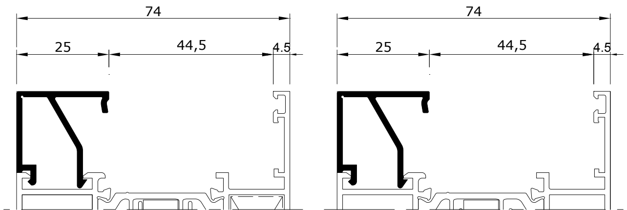
EX 50025-15 0.346 kg/m
