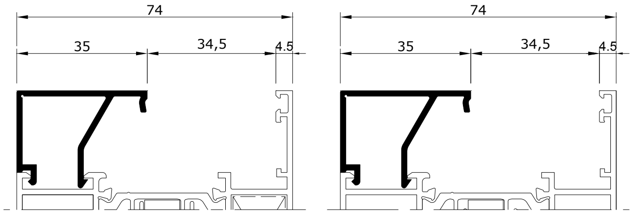
EX 50035-15 0.387 kg/m
